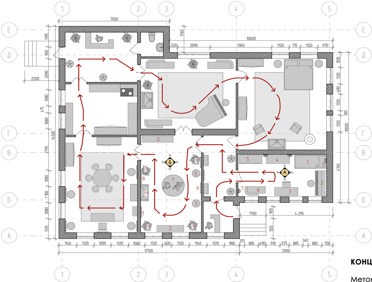
ПЛАН ІНТЕР'ЄРУ З ПОВЕРХУ МУЗЕЙНОГО ПРОСТОРУ М 1:50
