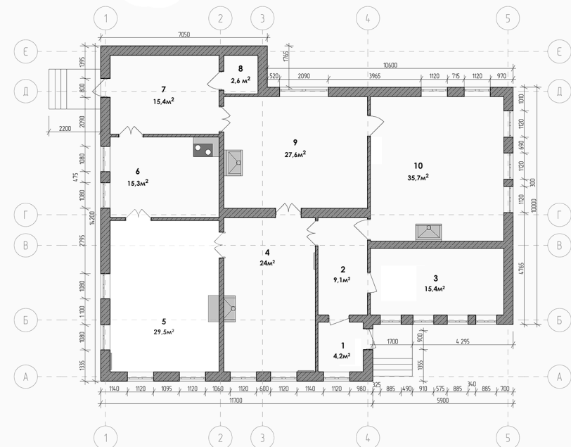
Обмірний план М 1:100
