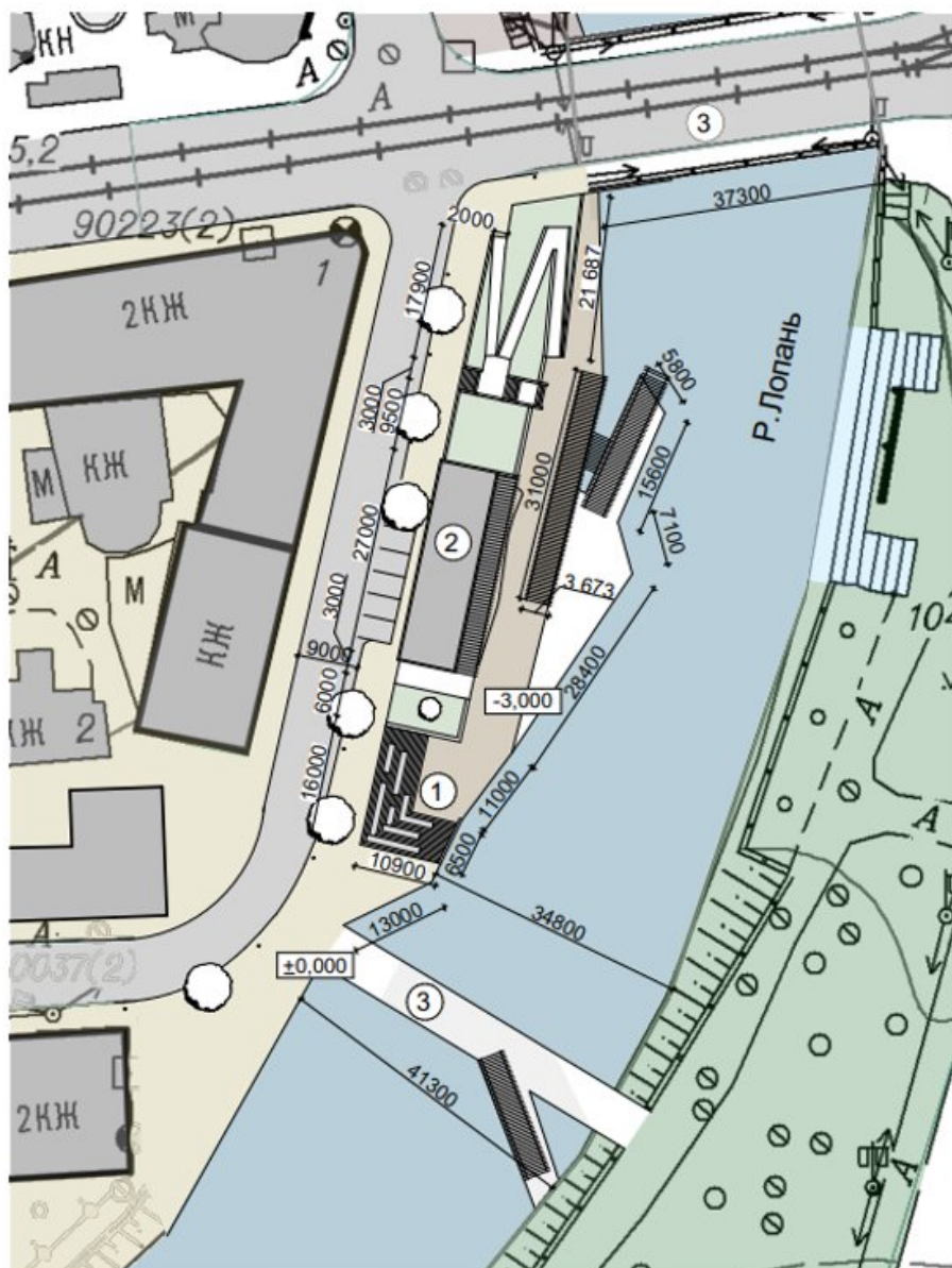
Генплан М 1:500
