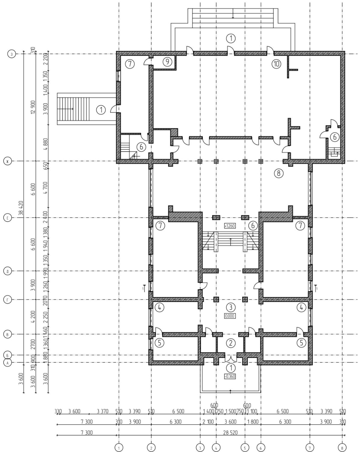
План першого поверху на відмітці +0.000 М 1:300
