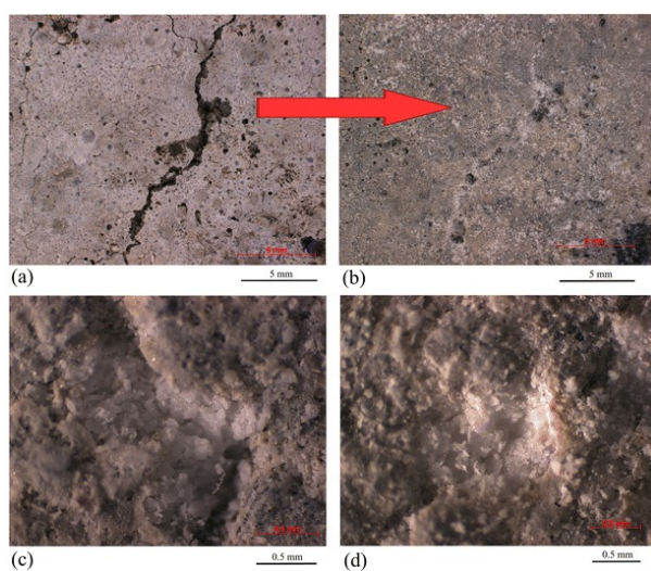
Іл. 29 - 30. Самовідновлюваний бетон та біодинамічний цемент. [42]
