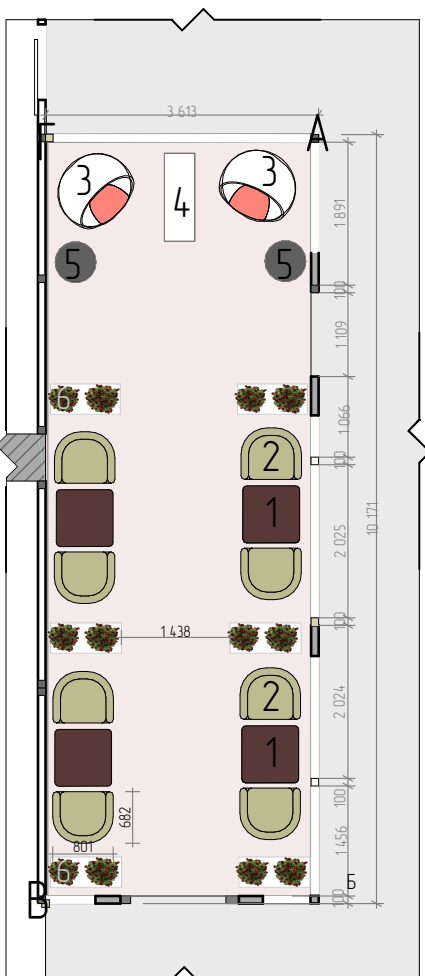
ПЛАН ПІДЛОГИ ВЕРАНДИ М 1:100
