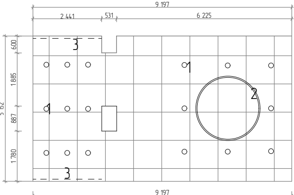
ПЛАН СТЕЛІ М ЛІНІЙНИЙ
