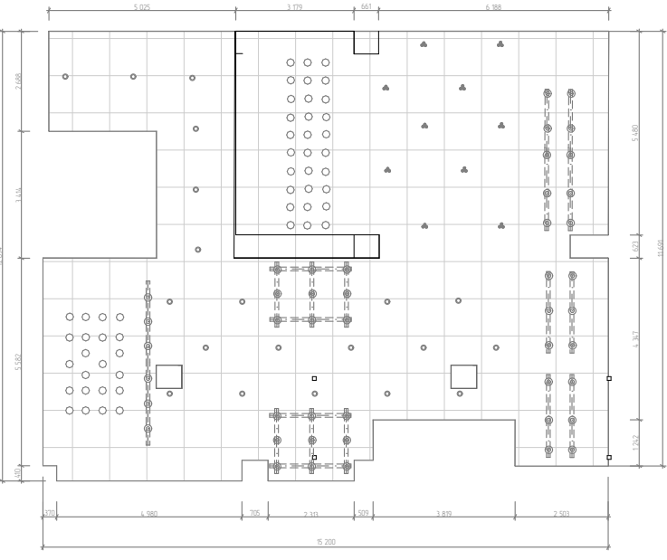
ПЛАН СТЕЛІ М.ЛІНІЙНИЙ
