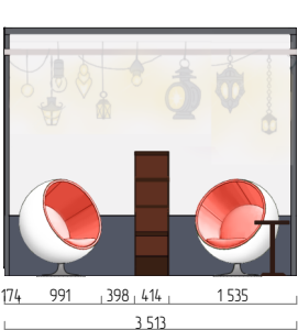
Розгортка ГА М 1:50
