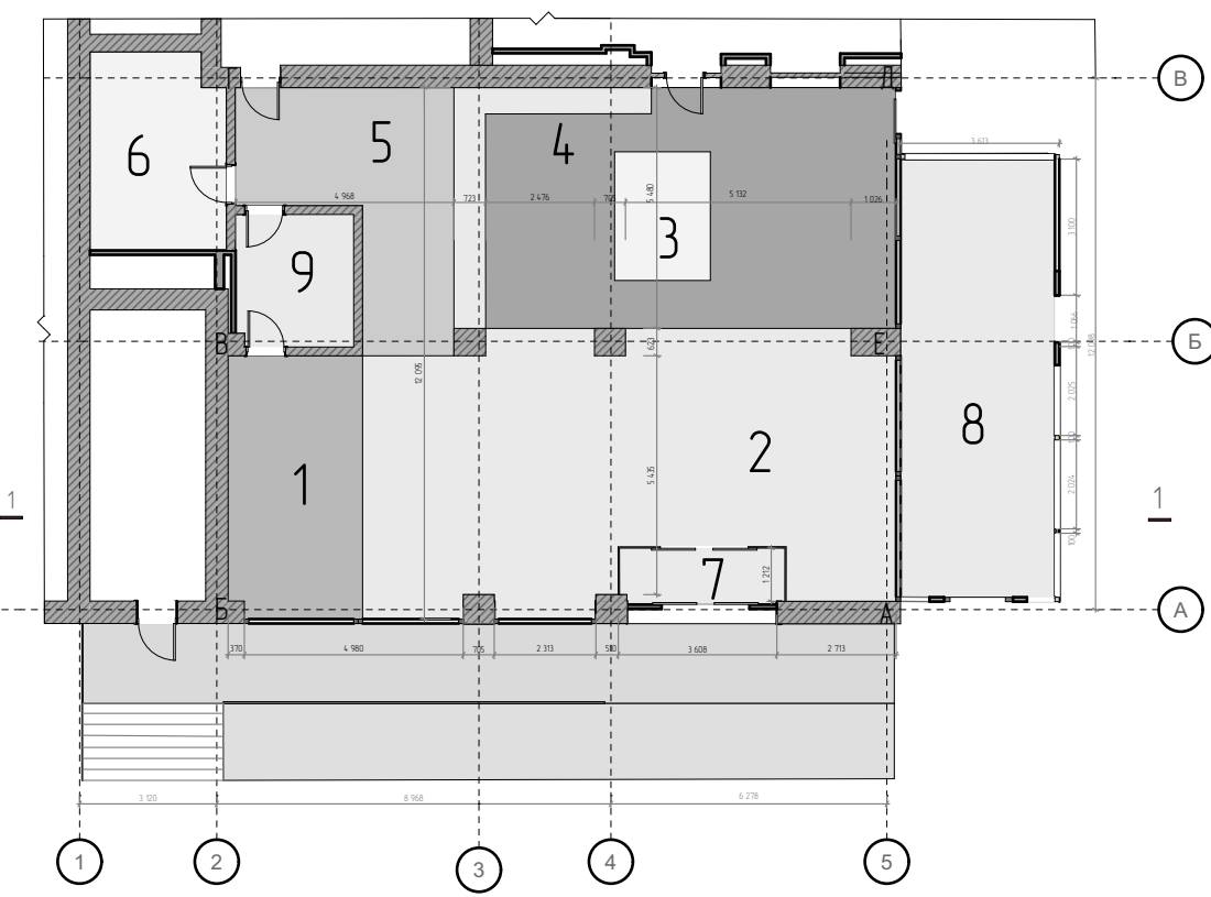
ПЛАН ПІДЛОГИ КІМНАТИ ДЛЯ ЗУСТРІЧЕЙ М 1:100
