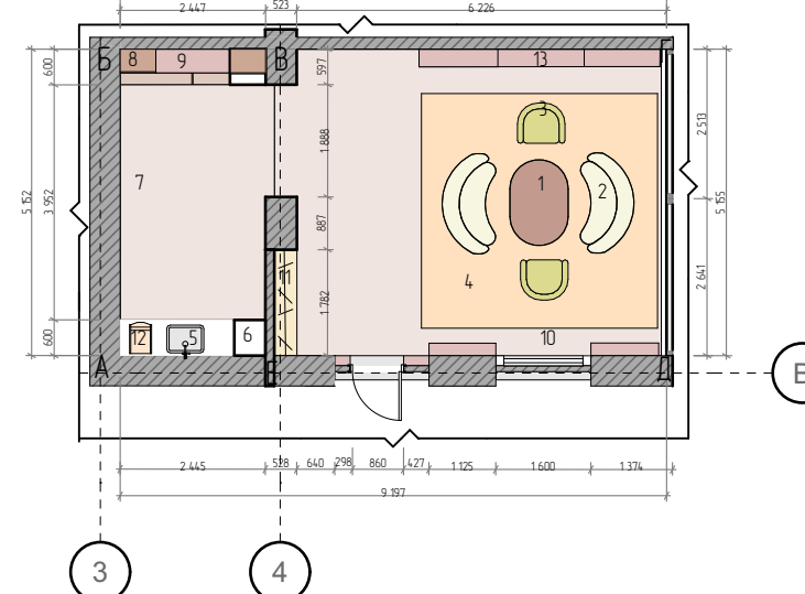
ПЛАН ПІДЛОГИ КІМНАТИ ДЛЯ ЗУСТРІЧЕЙ М 1:100
