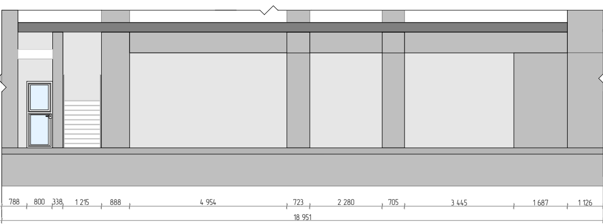
ФРАГМЕНТ РОЗРІЗУ М 1:120
