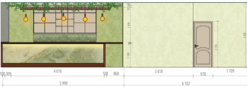
Розгортка БГ М 1:100
