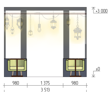
Розгортка БВ М 1:150
