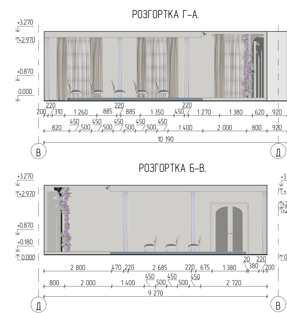
РОЗГОРТКИ ПРИМІЩЕННЯ ДРАЦСУ. М. ЛІНІЙНИЙ 0 1 2 3
