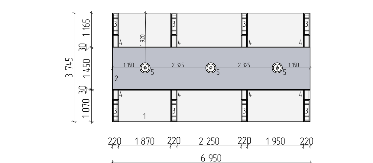
ПЛАН СТЕЛІ КІМНАТИ ОЧІКУВАННЯ. М. ЛІНІЙНИЙ 0 1 2 3
