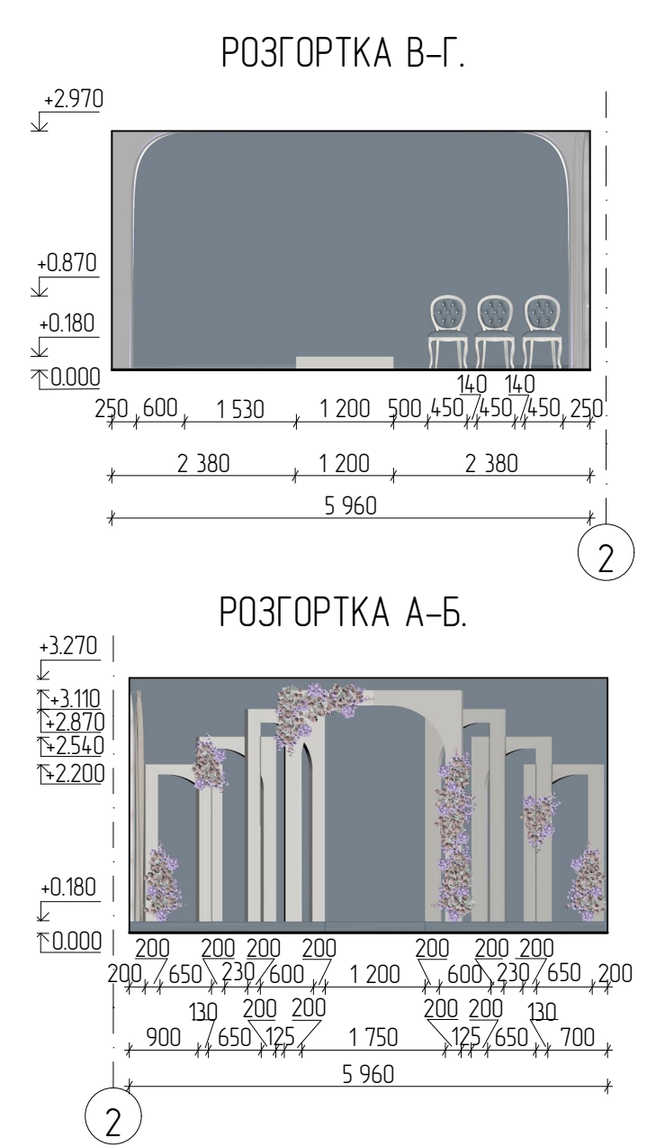
РОЗГОРТКИ ПРИМІЩЕННЯ ДРАЦСУ. М. ЛІНІЙНИЙ 0 1 2 3
