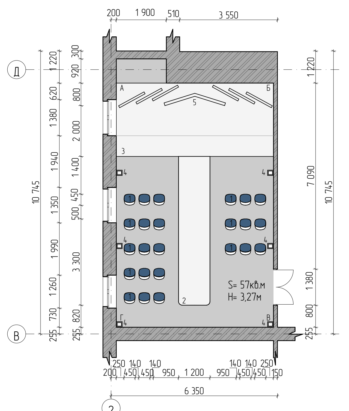
ПЛАН ПІДЛОГИ ДРАЦСУ. ВАРІАНТ 1. М. ЛІНІЙНИЙ 0 1 2 3
