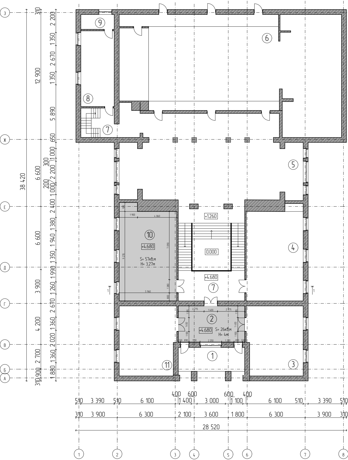
ПЛАН ДРУГОГО ПОВЕРХУ НА ВІДМІТЦІ +4.680 М 1:200
