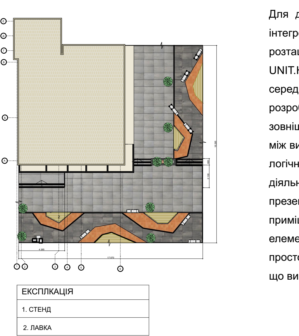
ПЛАН ВУЛИЧНА ВИСТАВКА М ЛІНІЙНИЙ
