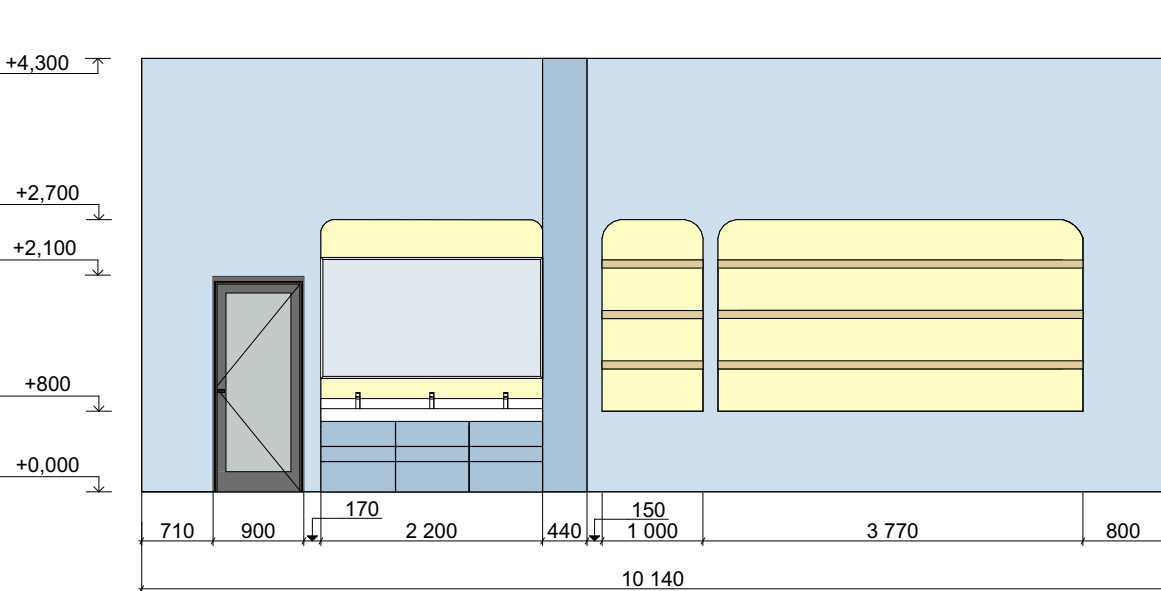
РОЗГОРТКА А-Б М 1:75
