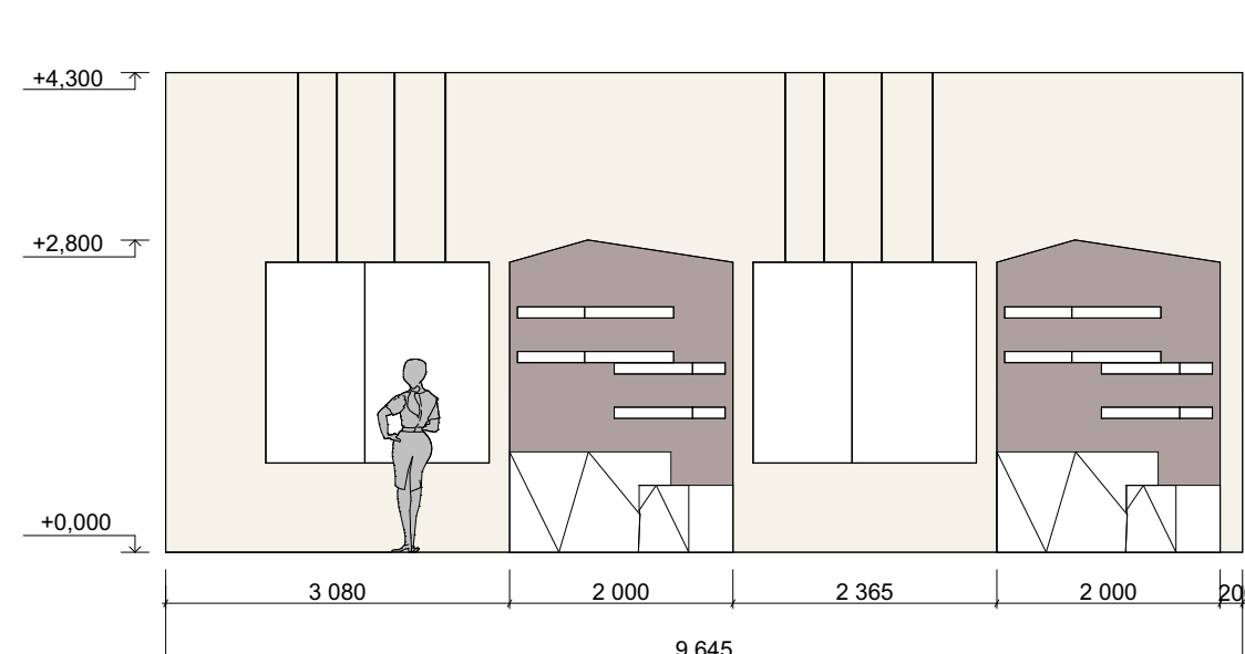
РОЗГОРТКА А-Б М 1:75
