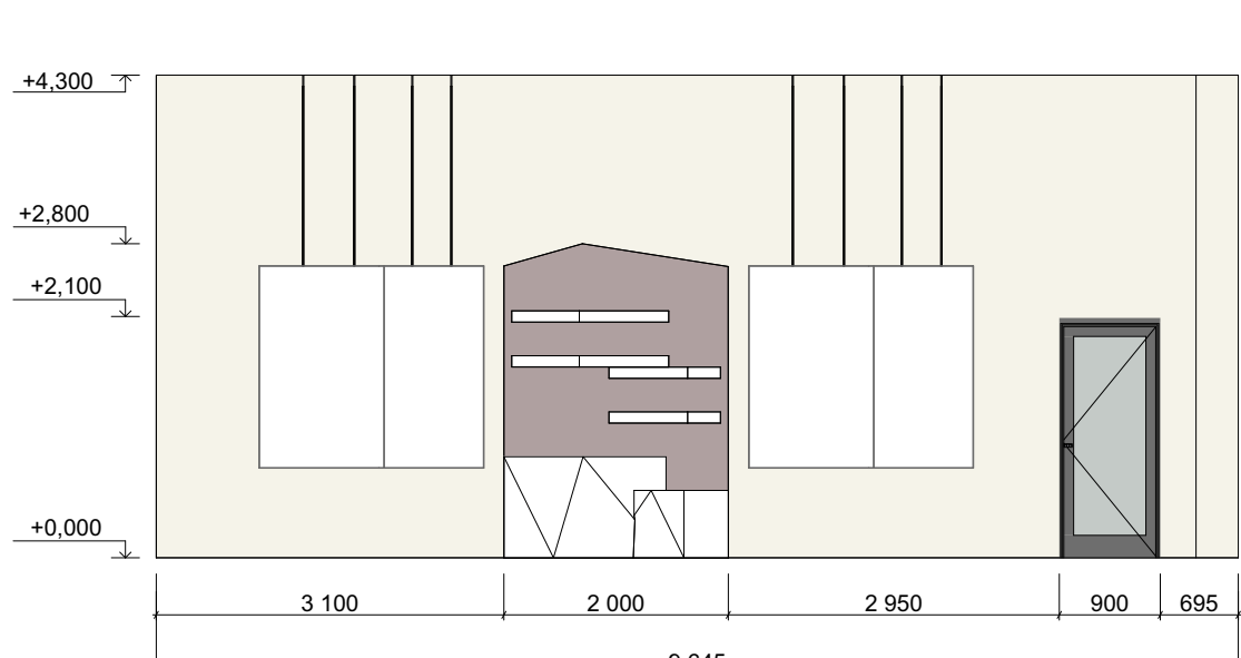
РОЗГОРТКА В-Г М 1:75
