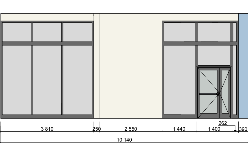
РОЗГОРТКА В-Г М 1:75
