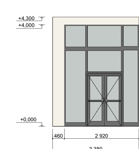
РОЗГОРТКА Г-А М 1:75
