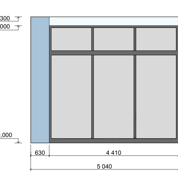
РОЗГОРТКА Г-А М 1:75
