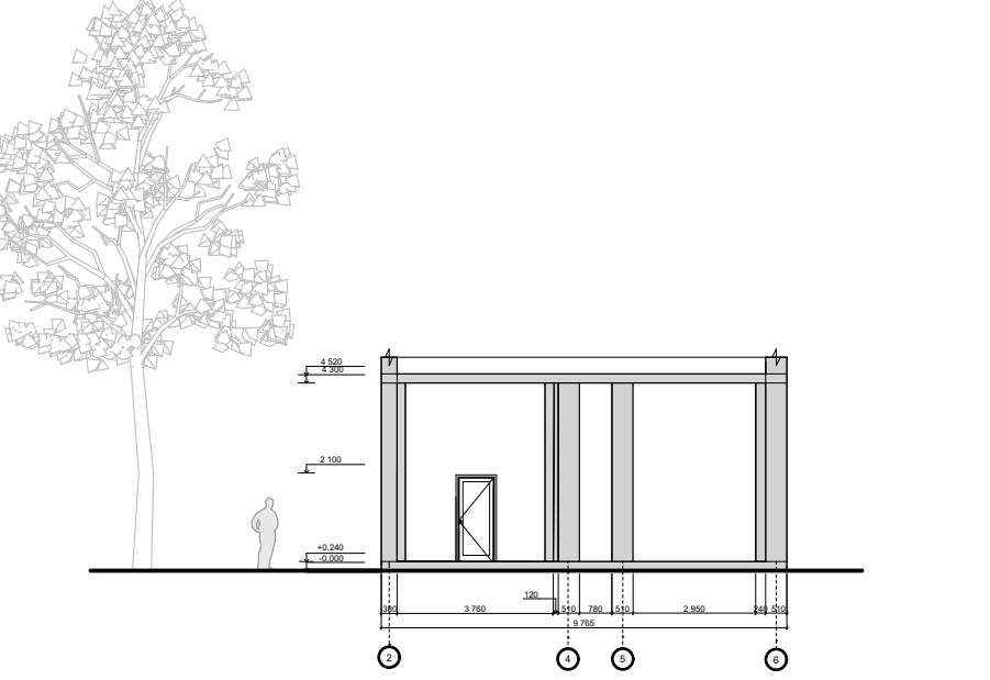
ФРАГМЕНТ РОЗРІЗУ 1-1 М 1:100
