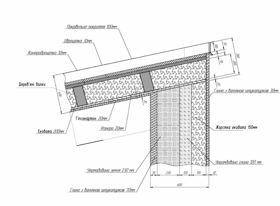
КОНСТРУКТИВНИЙ ВУЗОЛ
