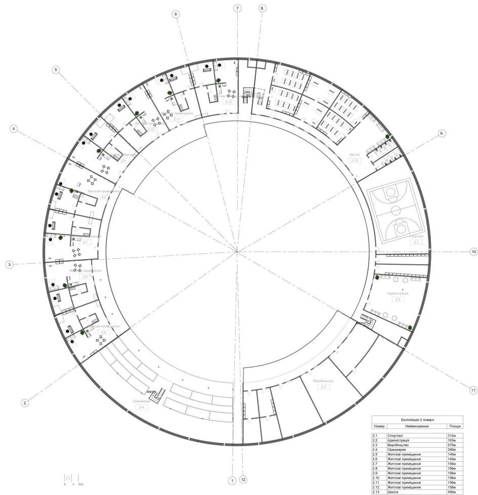
ПЛАН 2 ПОВЕРХУ М 1:200
