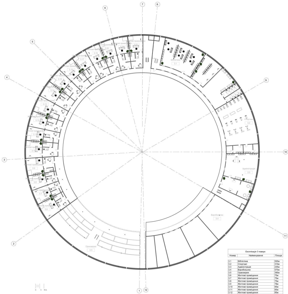
ПЛАН 3 ПОВЕРХУ М 1:200
