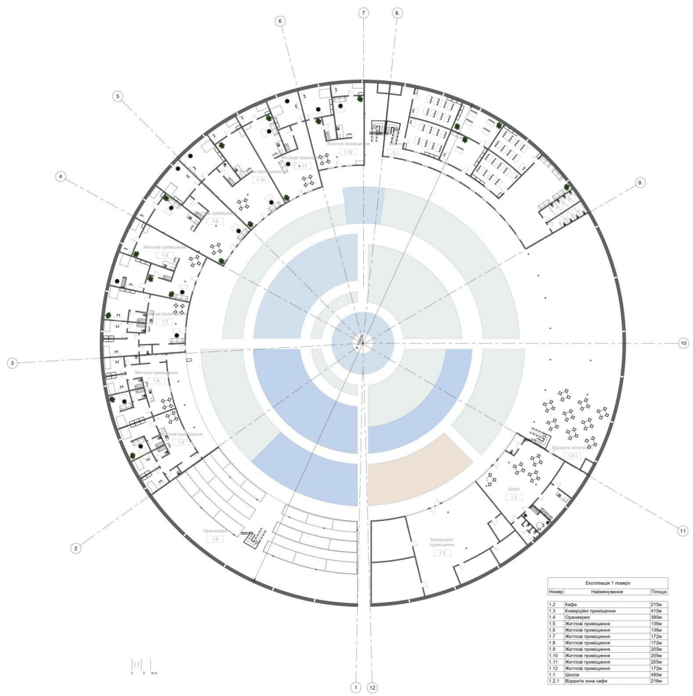
ПЛАН 1 ПОВЕРХУ М 1:200
