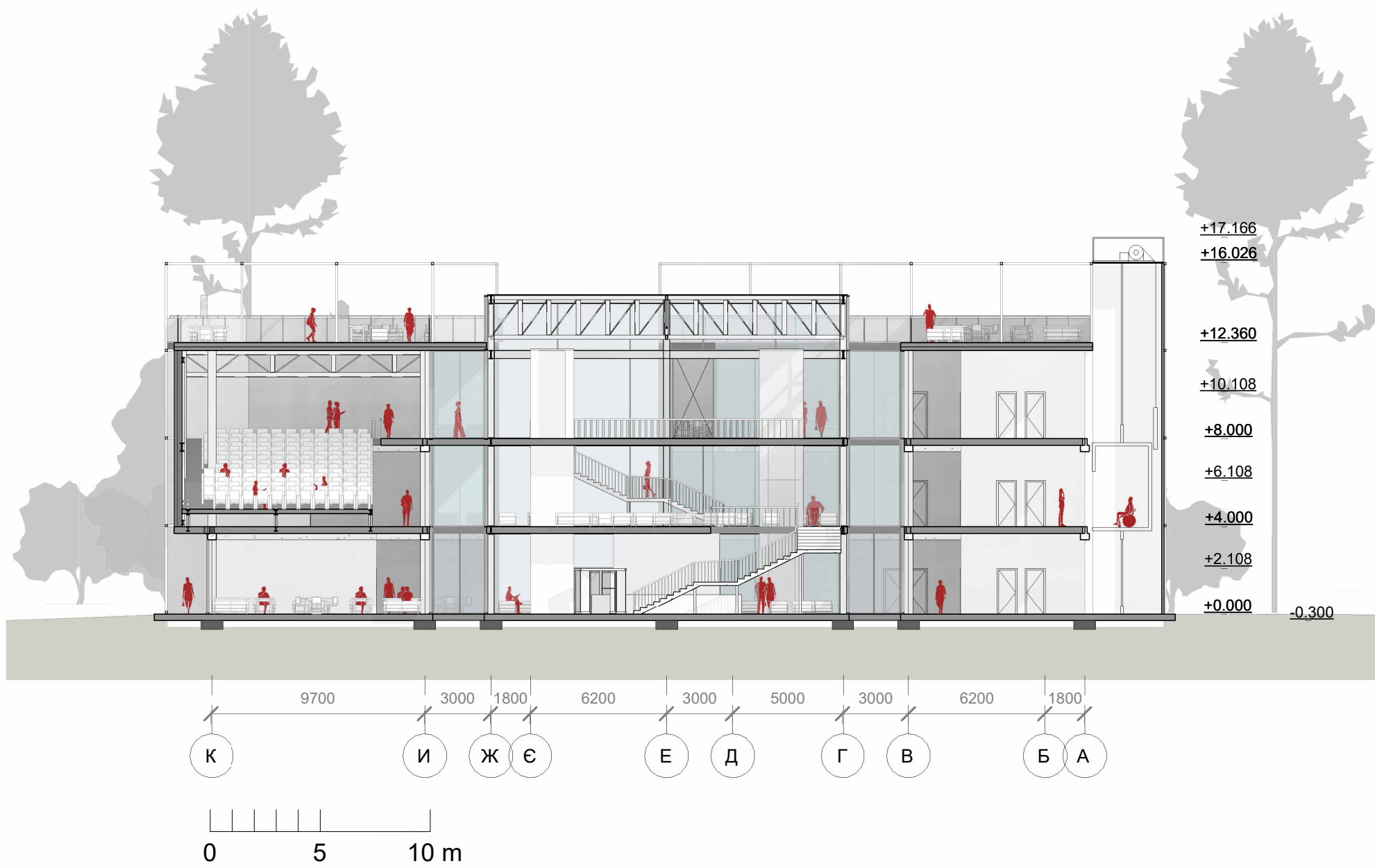
Розріз 3-3
