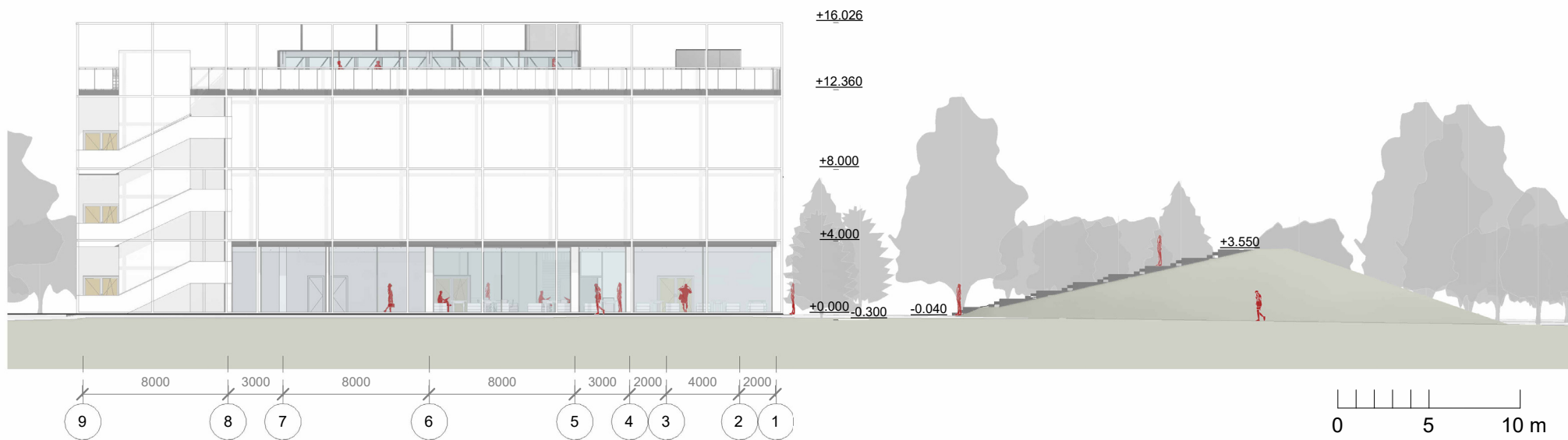
Фасад в вісях 9-1 Фасад в вісях 1-9
