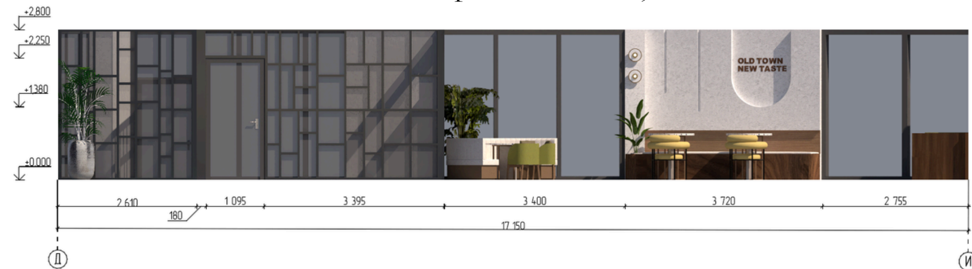
Розгортка Д-И М 1:50
