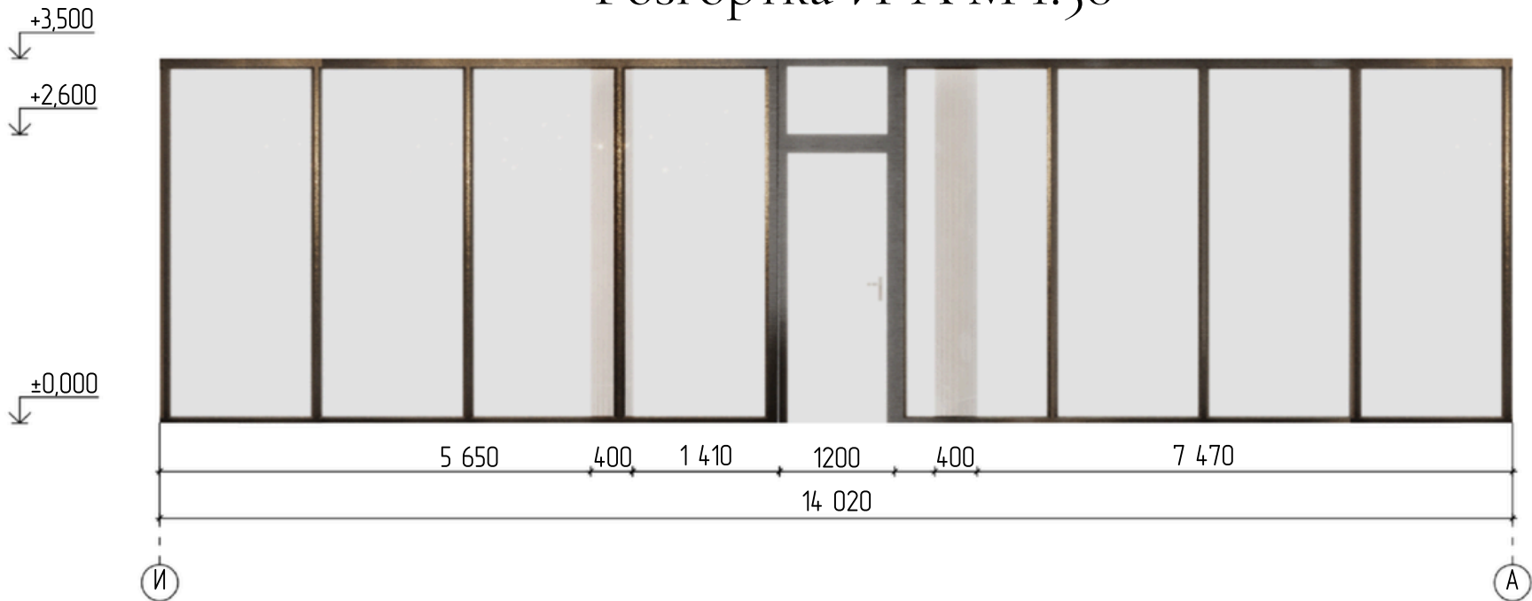
Розгортка И-А М 1:50
