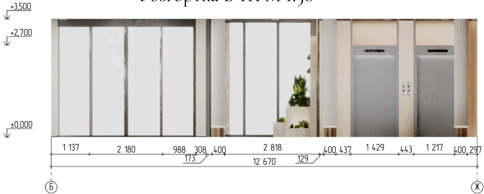
Розгортка Б-Ж М 1:50
