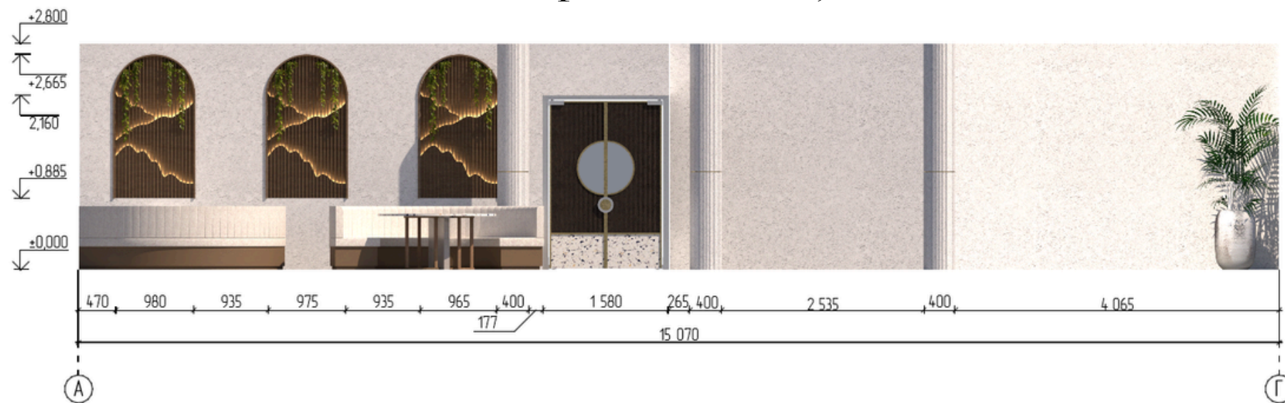
Розгортка А-Г М 1:50
