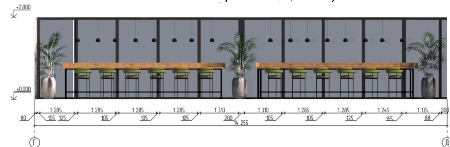
Розгортка Г-Д М 1:50
