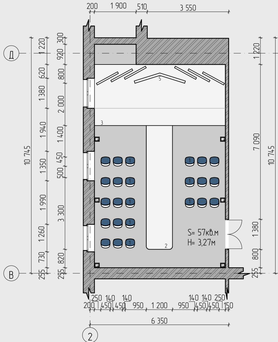
План підлоги М 1:100. Варіант 1
