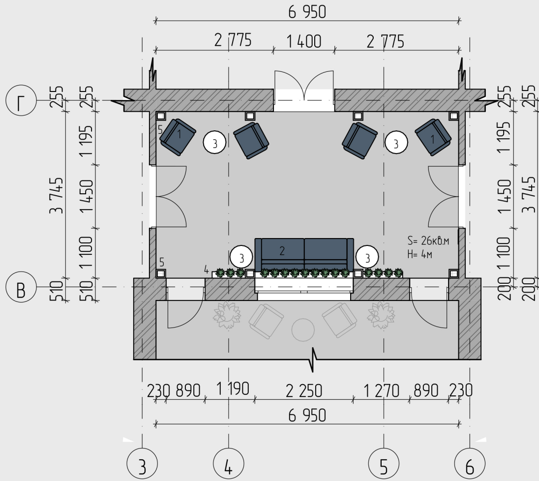
План підлоги М Лінійний 0 1 2 3
