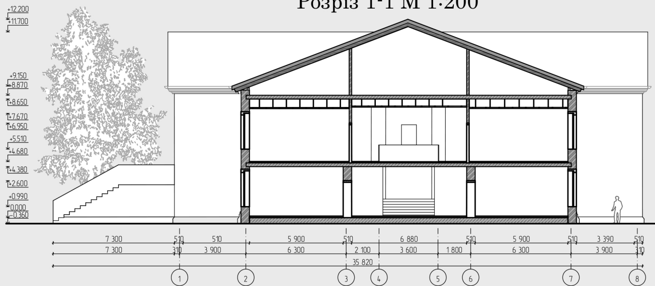
Розріз 1-1 М 1:200
