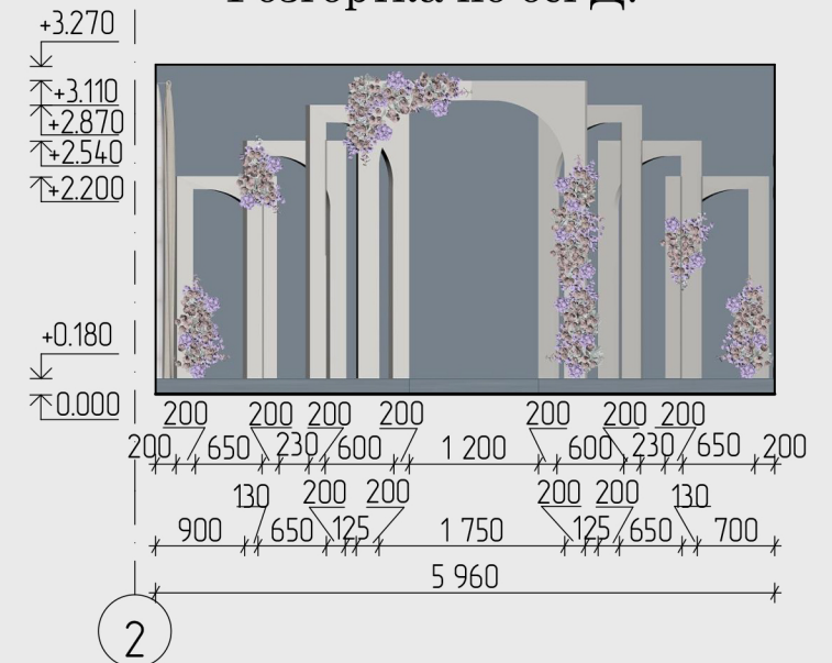
Розгортка по осі Д.
