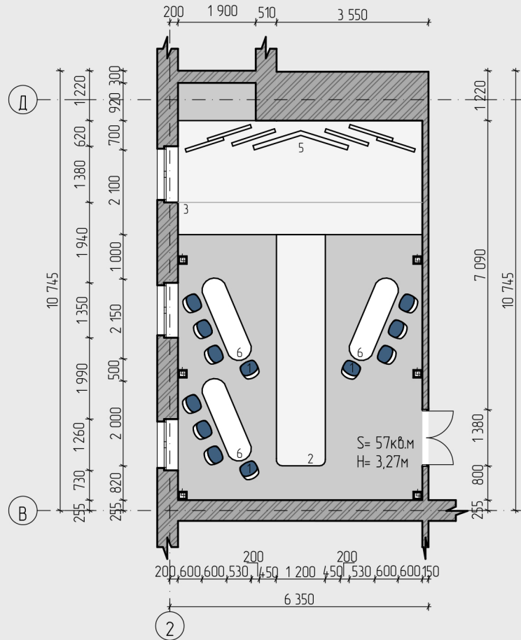
План підлоги М Лінійний 0 1 3 4 Варіант 2
