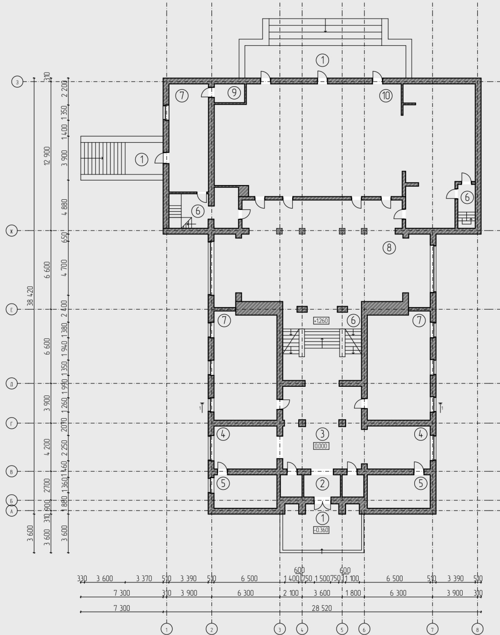
План першого поверху на відмітці +0.000 М 1:300
