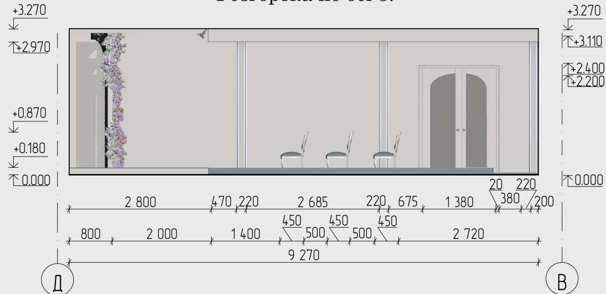
Розгортка по осі 3.
