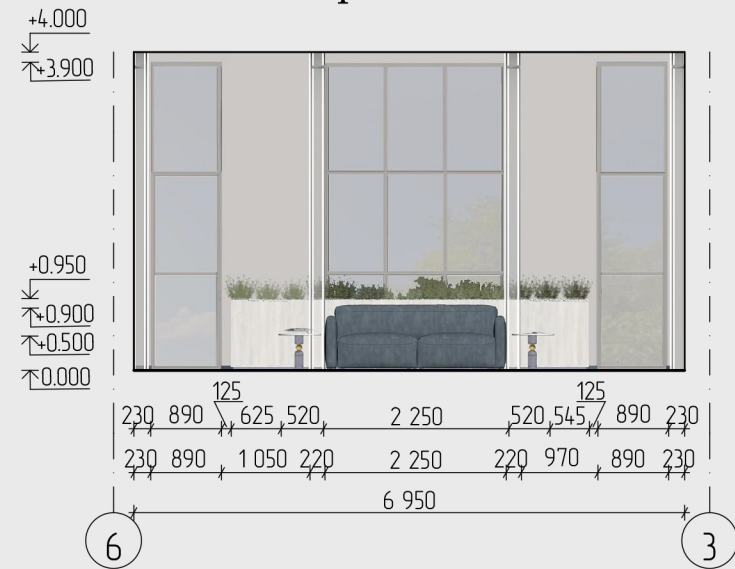
Розгортка по осі В.
