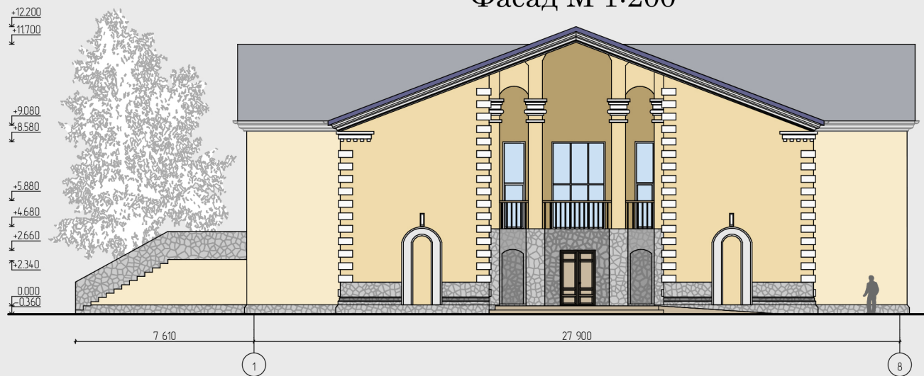
Фасад М 1:200
