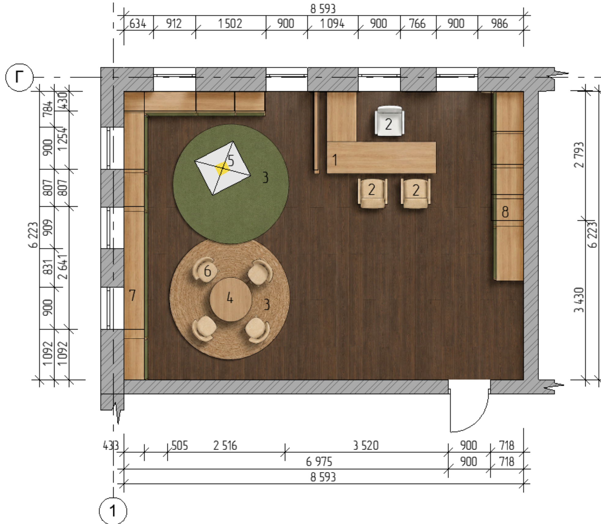
ПЛАН ПІДЛОГИ
