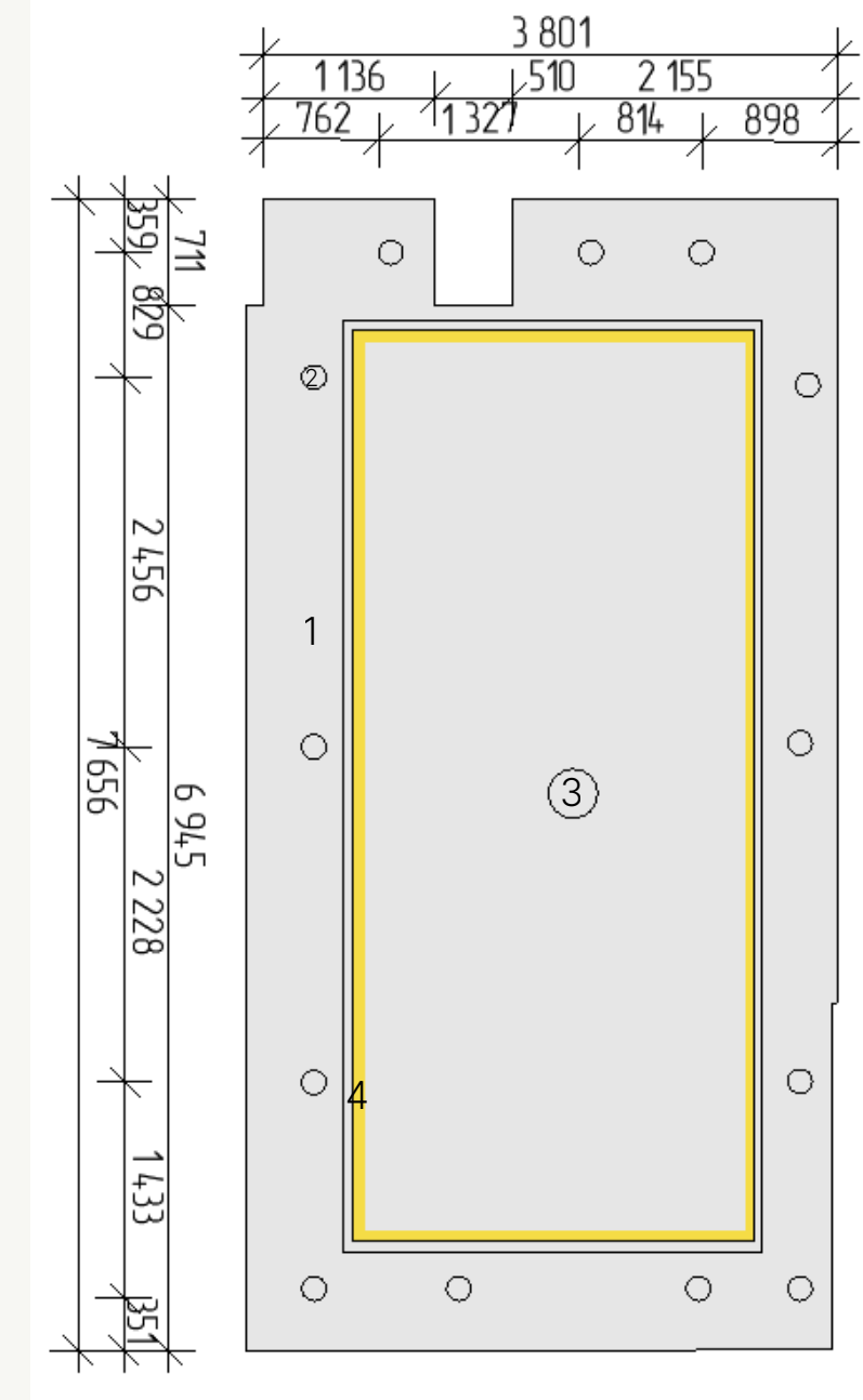
ПЛАН СТЕЛІ
