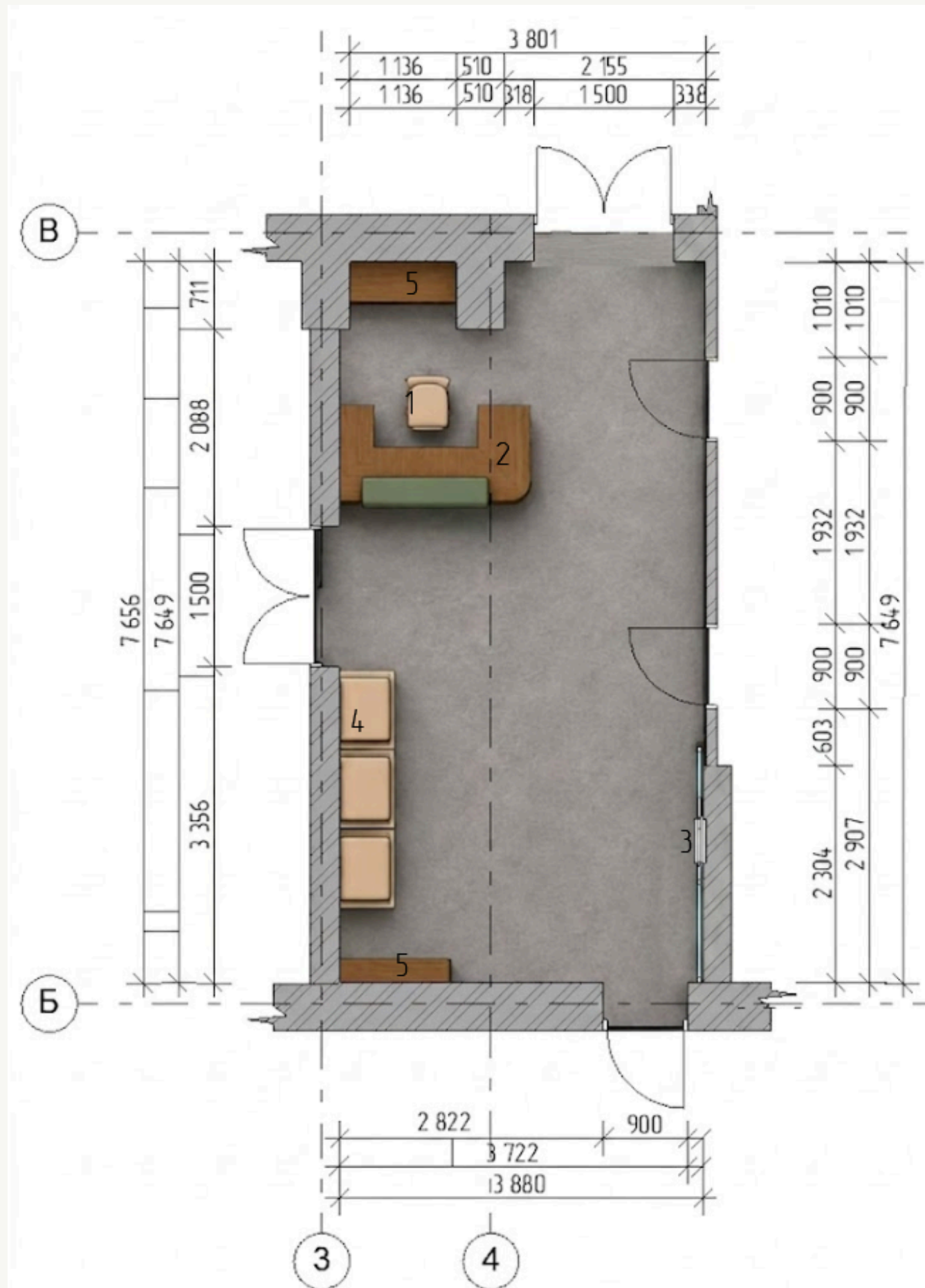
ПЛАН ПІДЛОГИ
