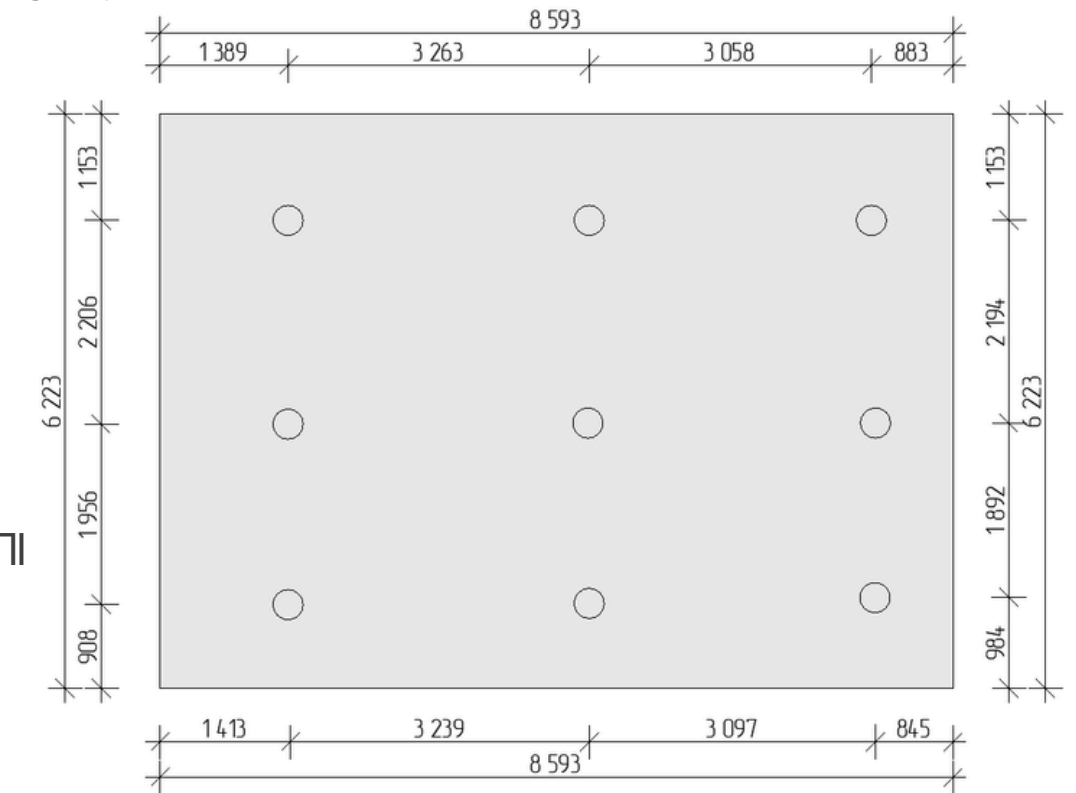
ПЛАН СТЕЛІ
