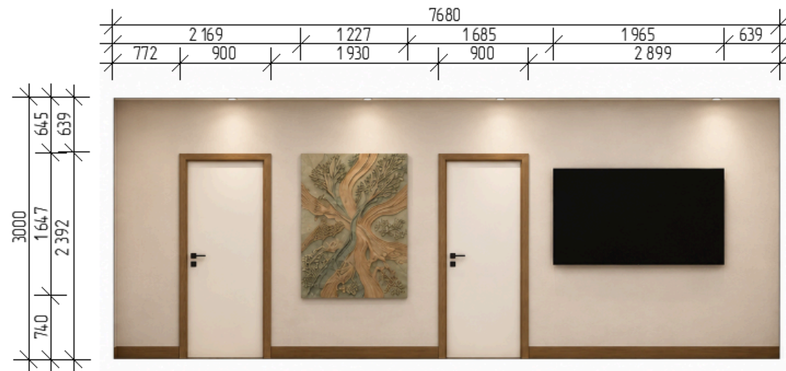
РОЗГОРТА СТІН ПО ОСІ 3
