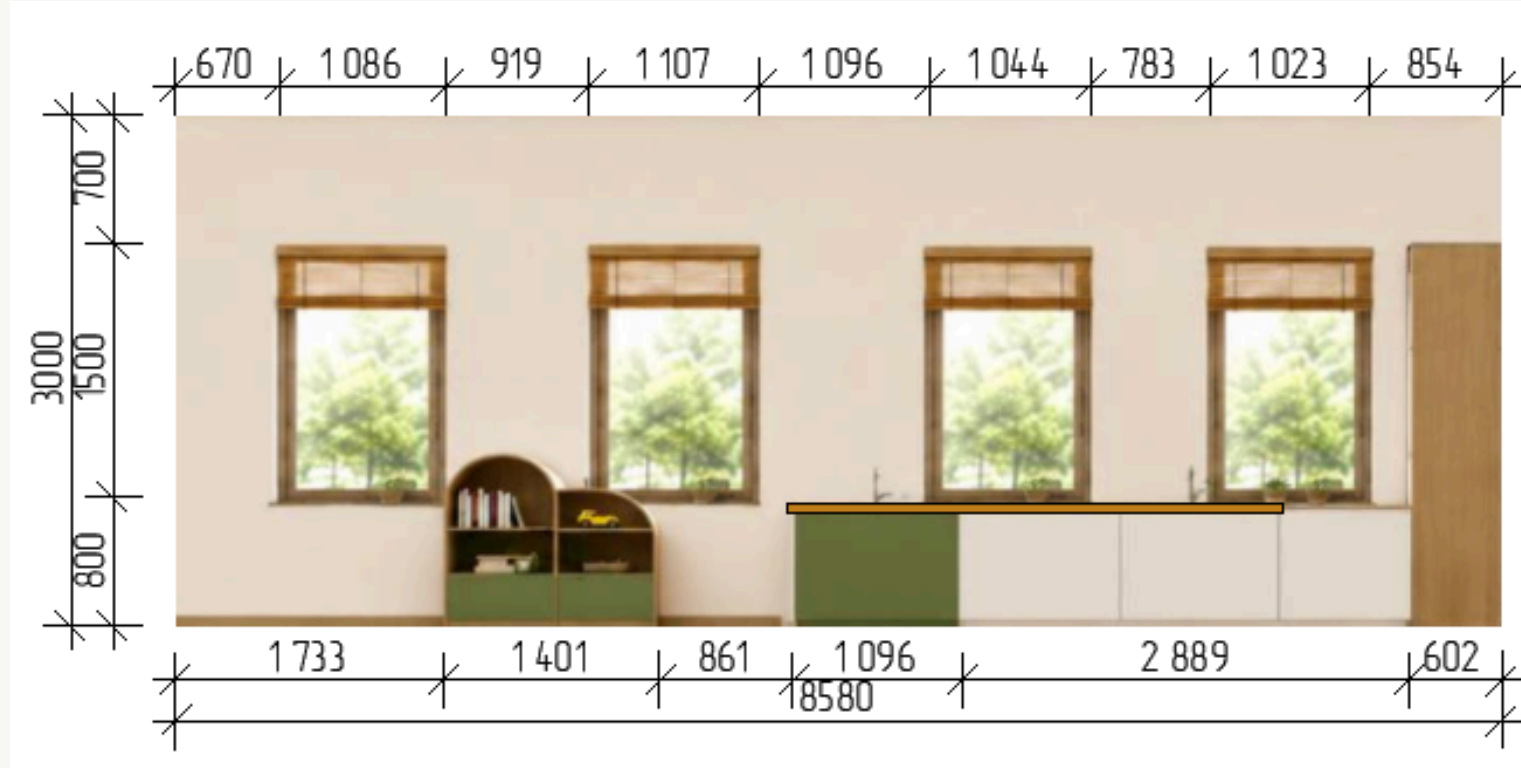
РОЗГОРТА СТІН ПО ОСІ Ф
