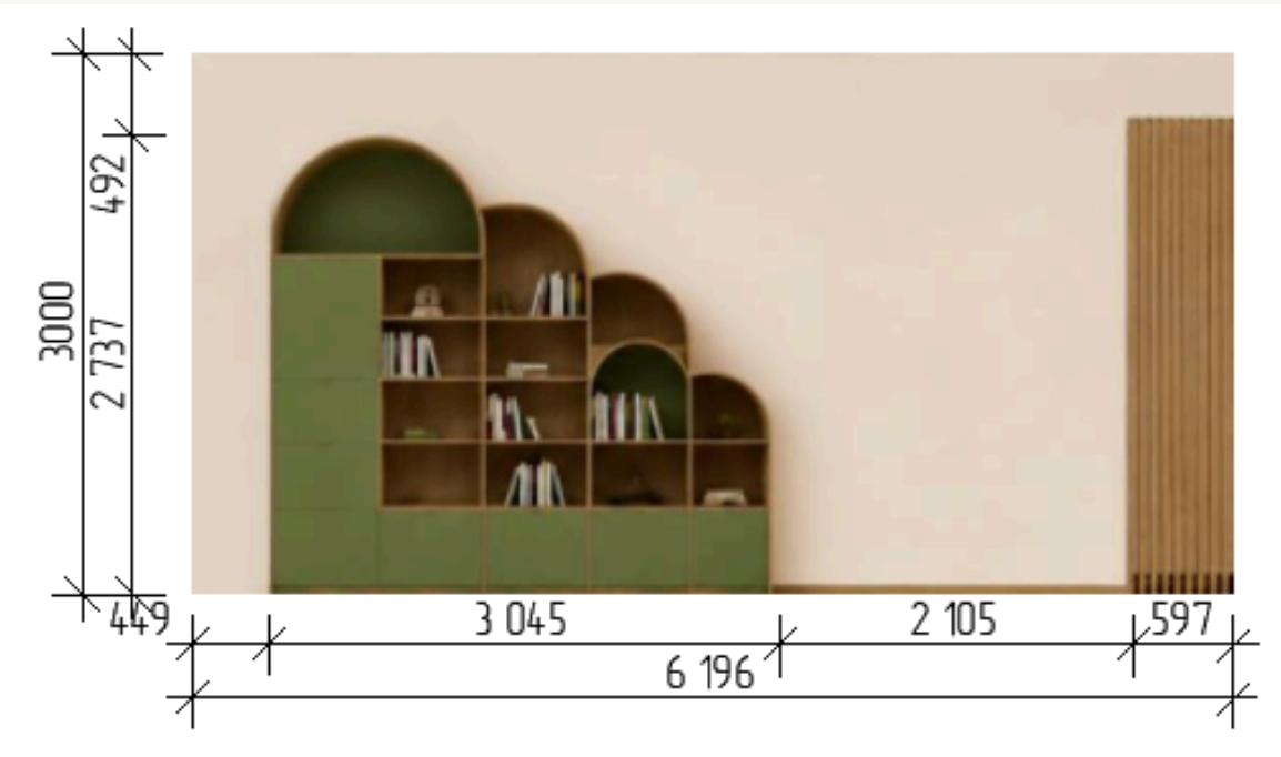
РОЗГОРТА СТІН ПО ОСІ П
