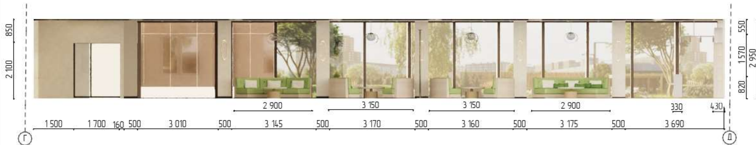
Розгортка по вісі 3 М 1:200
