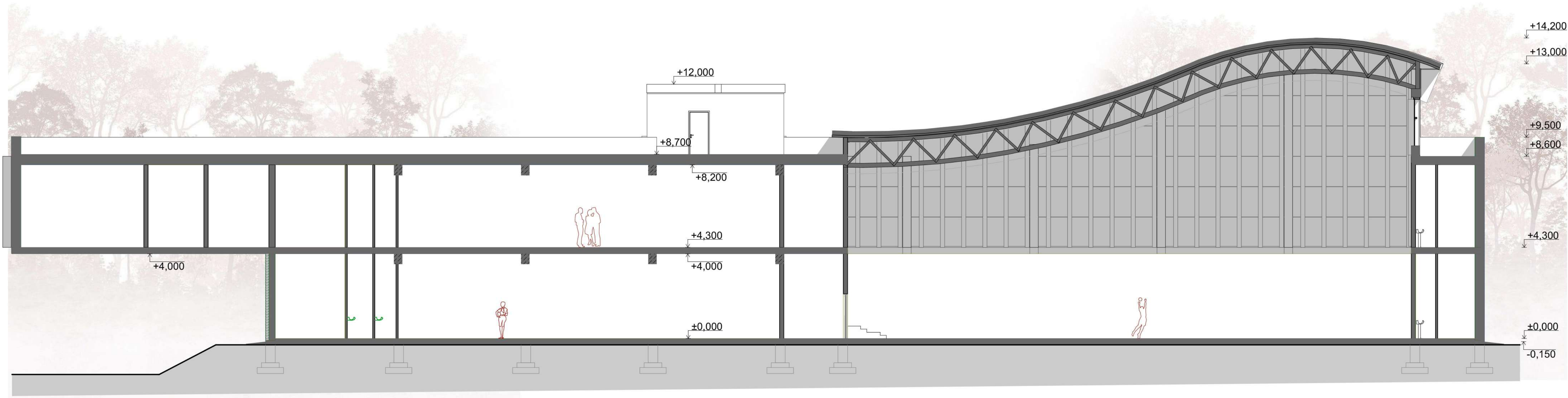
Розріз 1-1
