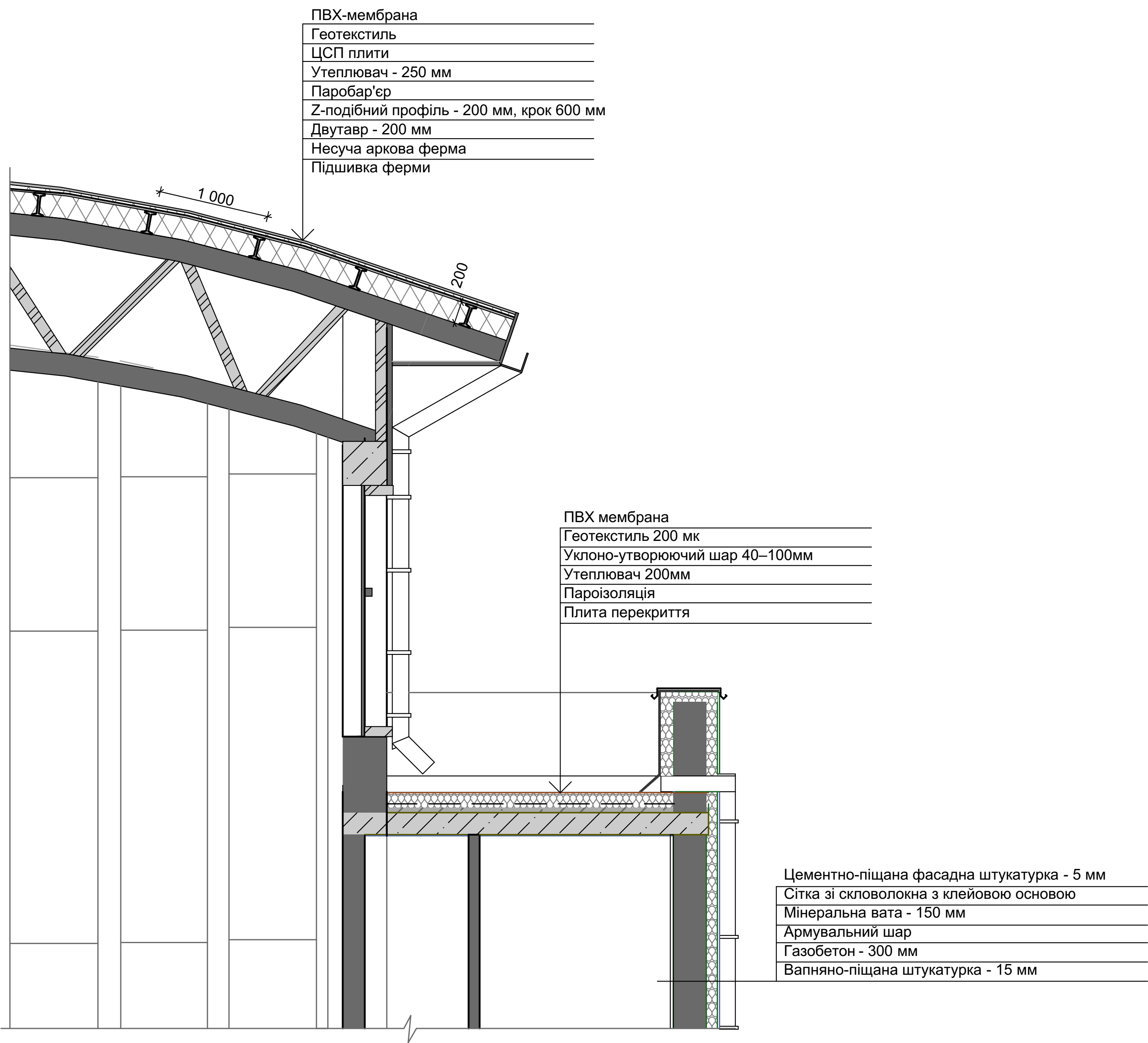
Конструктивний вузол
