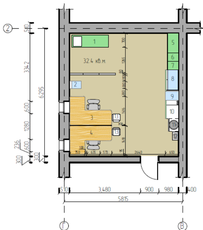
План підлоги кабінету сімейного лікаря М 1:150
