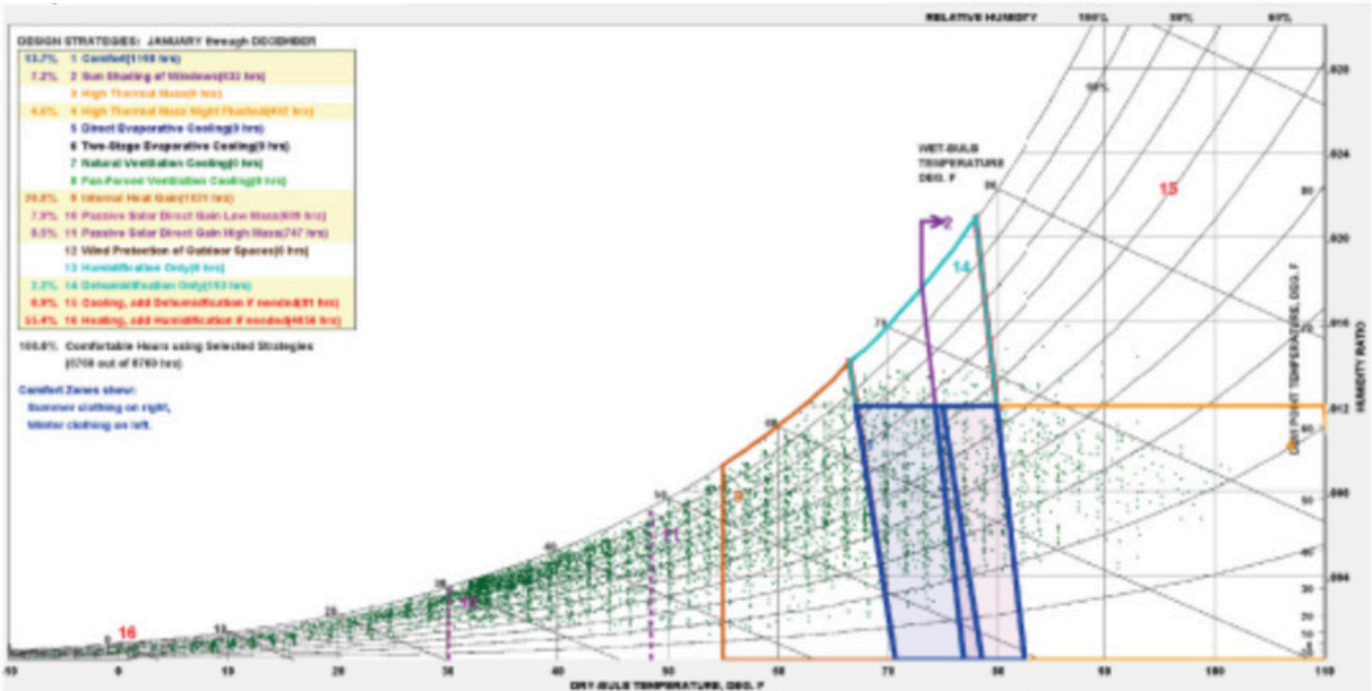
ПСИХОМЕТРИЧНА ДІАГРАМА/ PSYCHOMETRIC CHART
