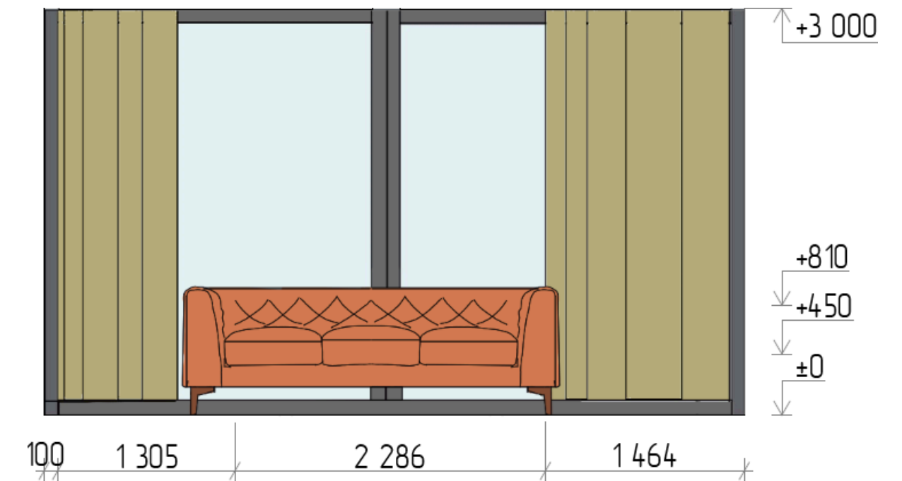
Розгортка ГА М 1:50
