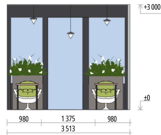
Розгортка БВ м 1:50
