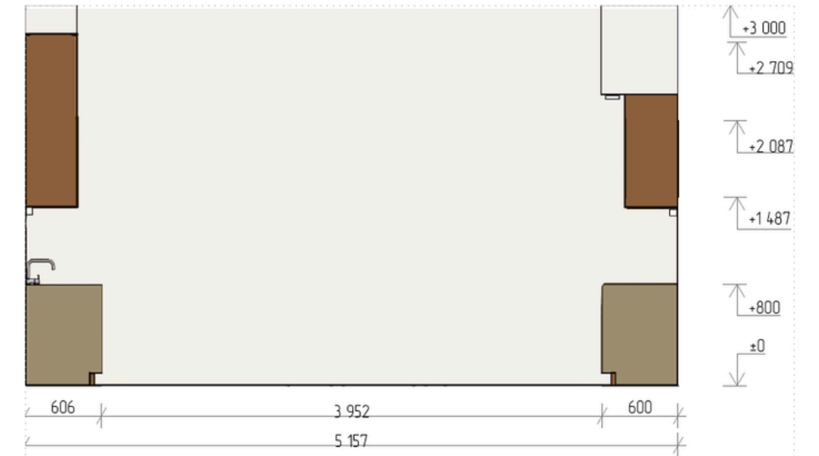
Розгортка ДА М 1:50
