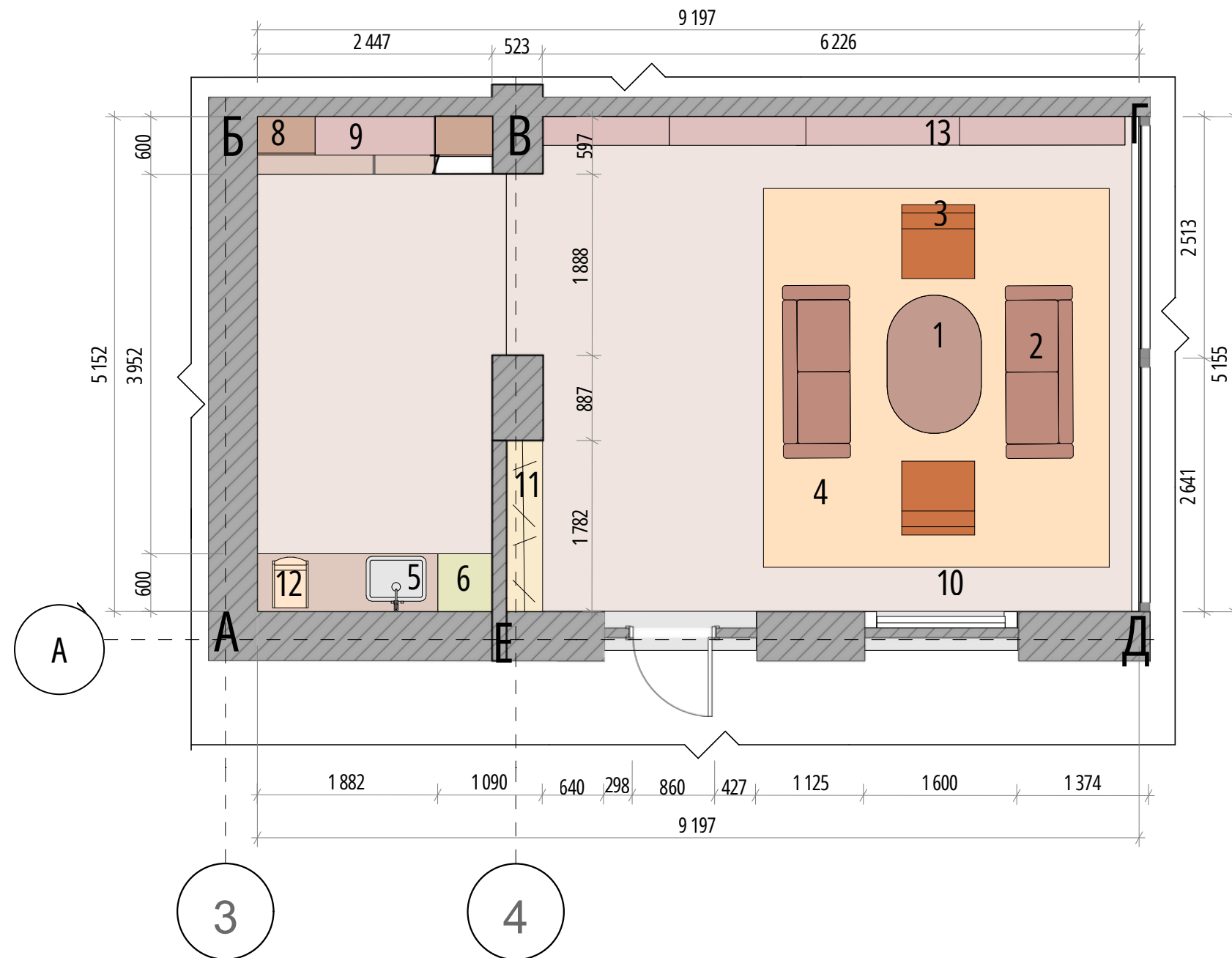
План підлоги м 1:50
