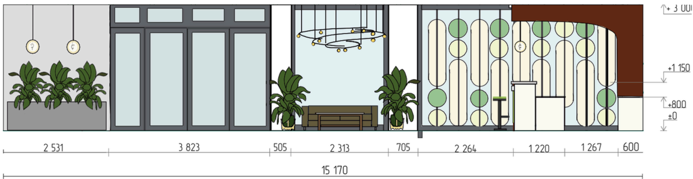
Розгортка А-Б м 1:50
