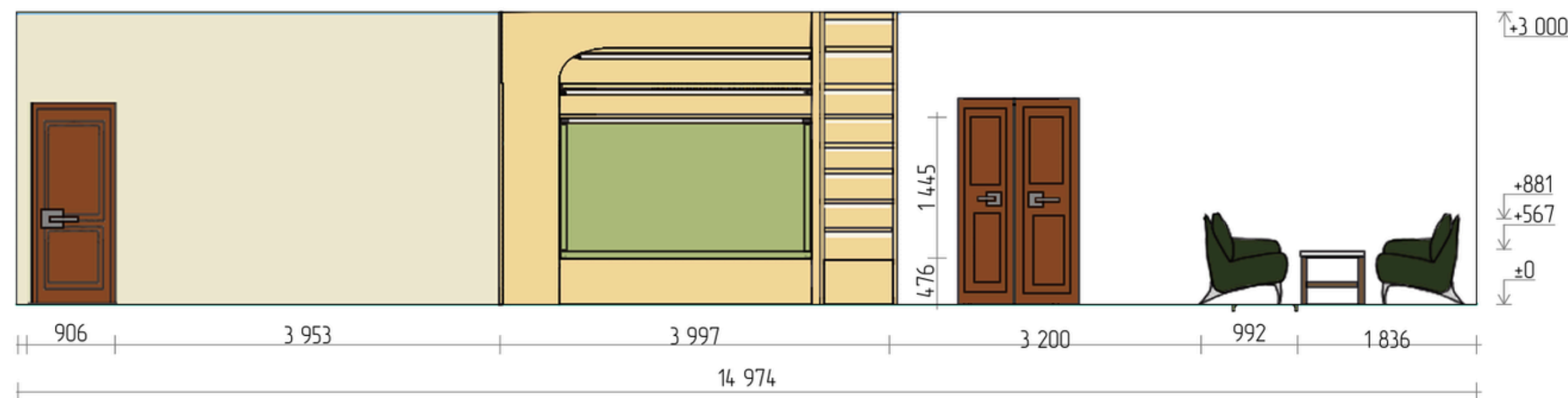
Розгортка А-Д м 1:50
