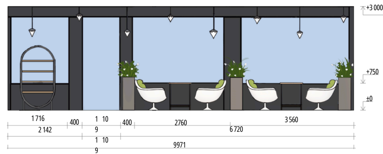
Розгортка БВ м 1:50
