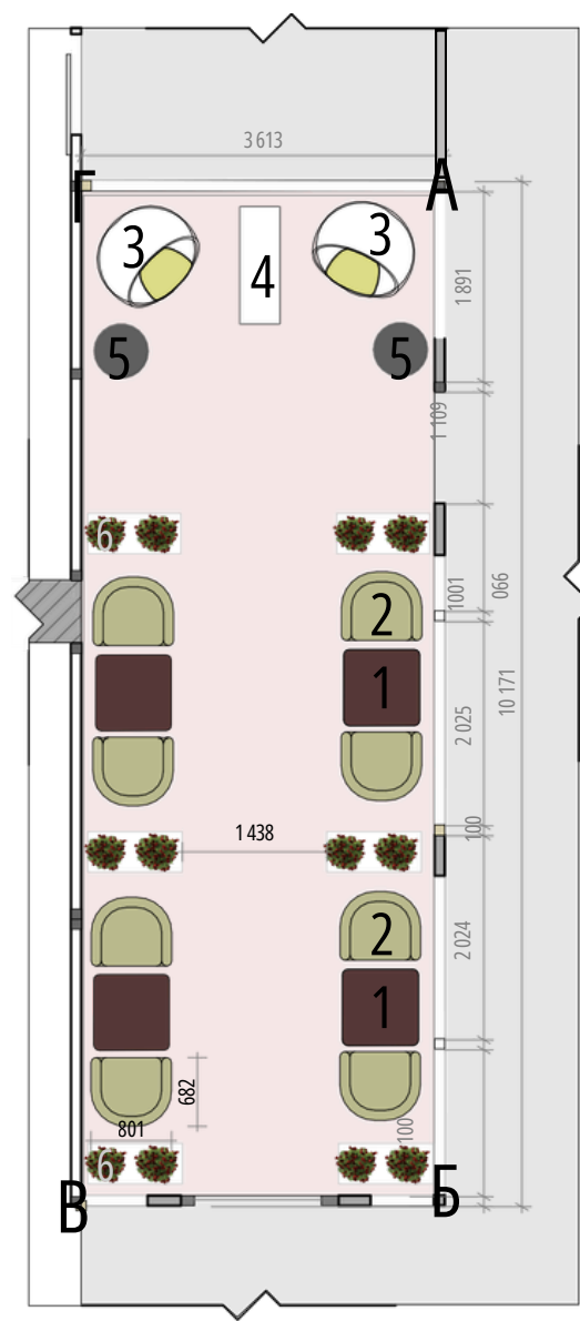
План підлоги м 1:50
