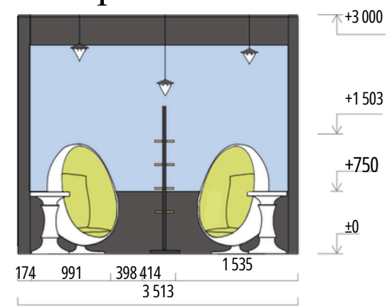
Розгортка ГА м 1:50
