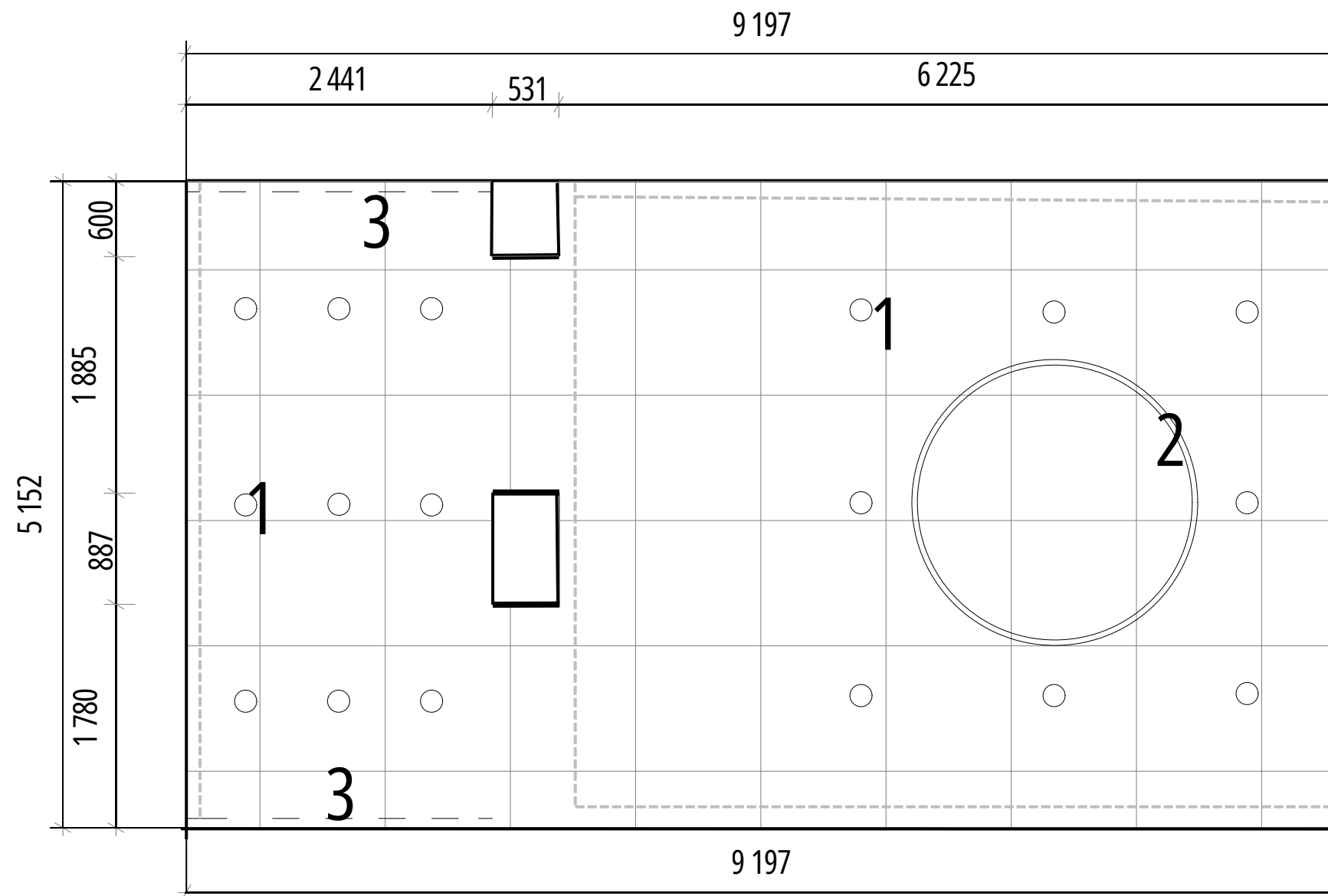
План стелі м 1:50
