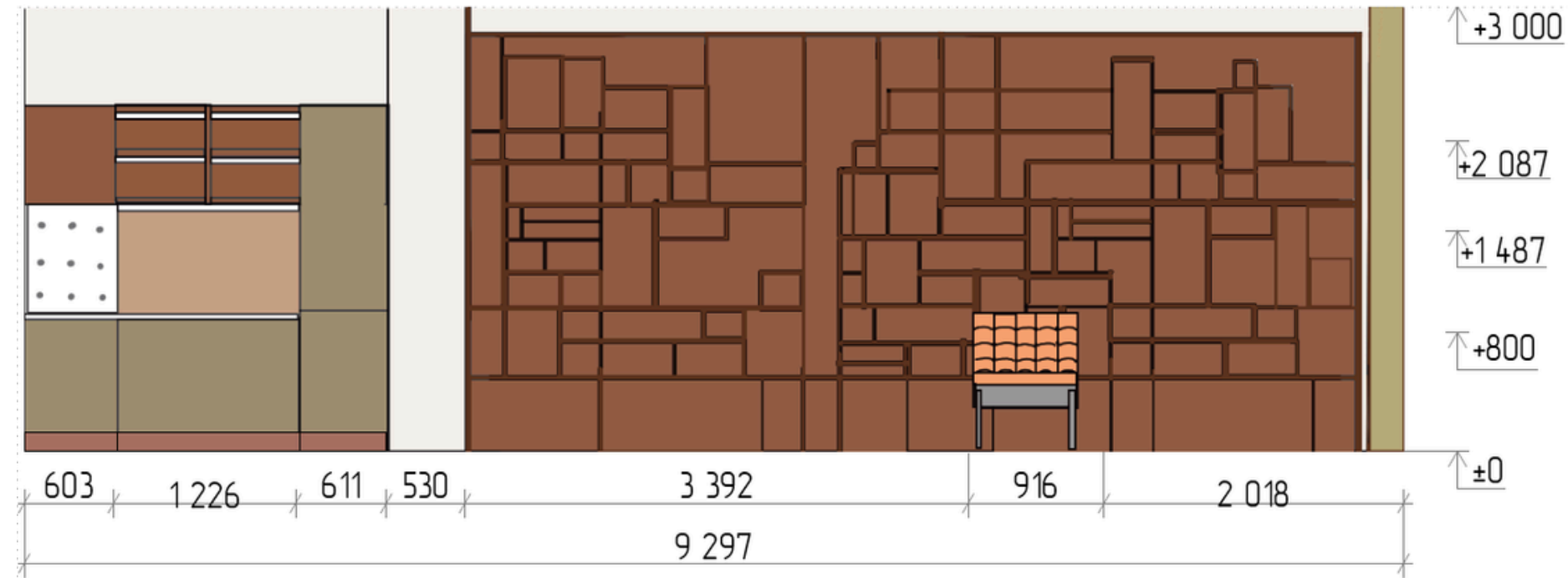
Розгортка БГ М 1:50
