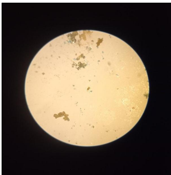
Іл. 95. Невідомий автор. “Марія здобула благодать у Бога”. Мікроскопічні дослідження, реакція авторського ґрунту з хлоридною кислотою. Фото Д. Е. Панової.
