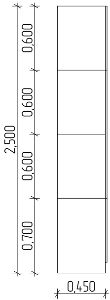
ВИД ЗБОКУ М 1:50
