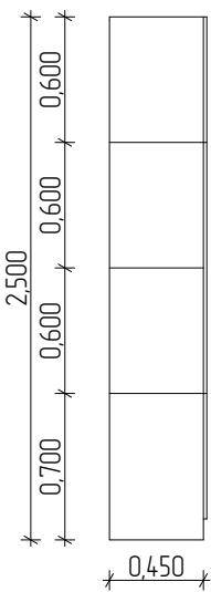
ВИД ЗБОКУ М 1:50
