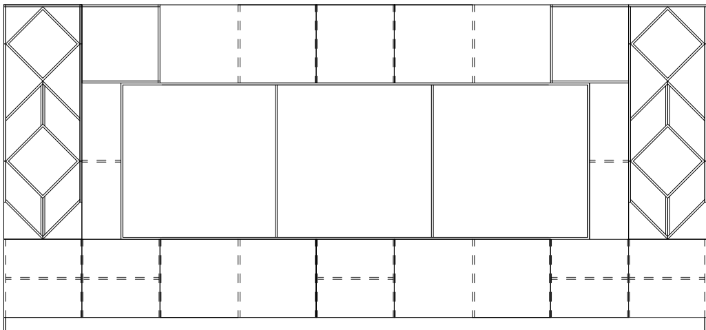
РОЗБИВКА НА ВНУТРІШНІ ПОЛИЦІ М 1:50
