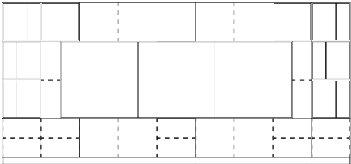
РОЗБИВКА НА ВНУТРІШНІ ПОЛИЦІ М 1:50
