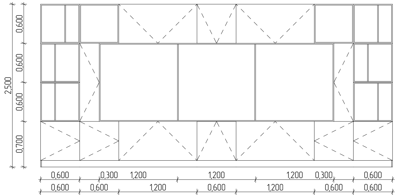
ВИД ЗПЕРЕДУ М 1:50
